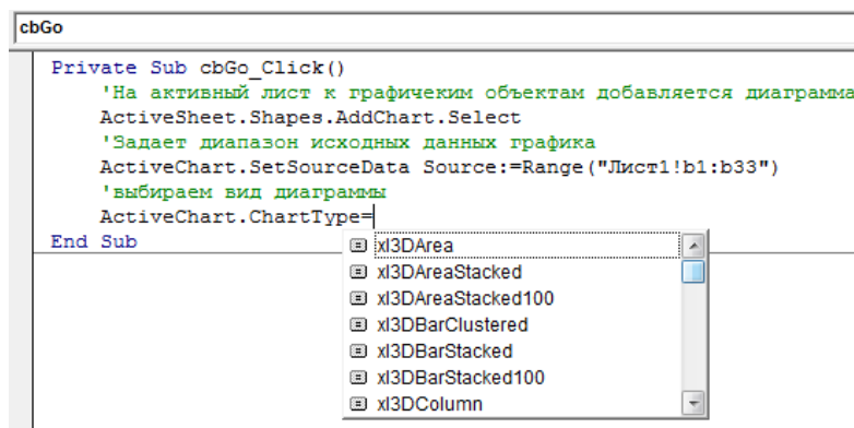
Рисунок 3.4 Изменение типа диаграммы
