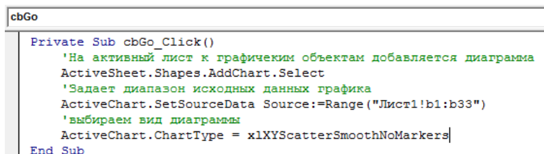
Рисунок 3.. 5 Изменение типа диаграммы на xlXYScatterSmoothNoMarkers
