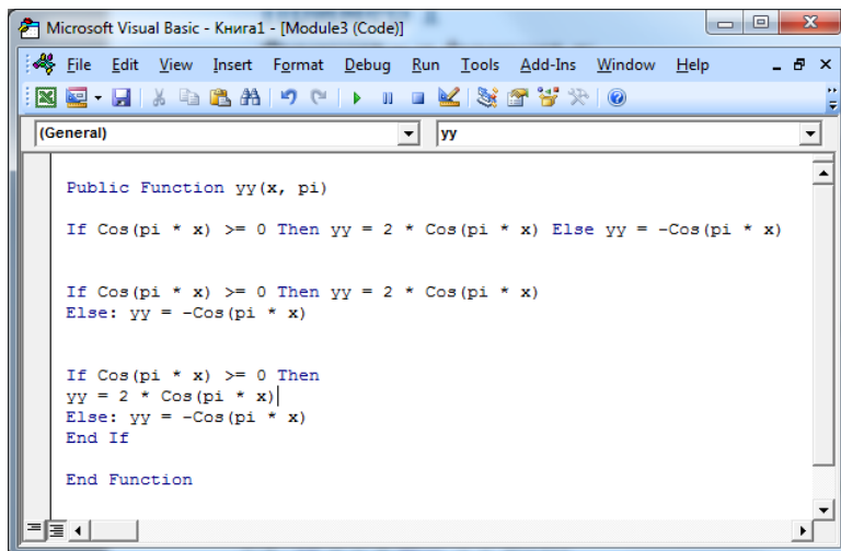
Рисунок 1.5. Создание пользовательской функции
