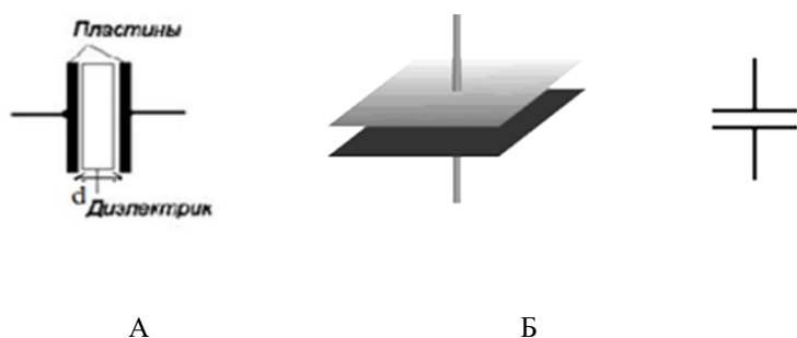
Рис. 20. Устройство плоского конденсатора (А, Б) и обозначение его на схеме (С)
