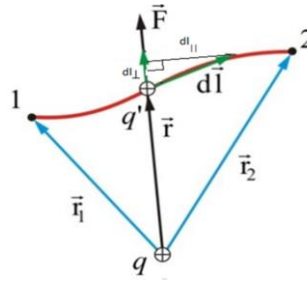
Рис. 9. Иллюстрация к доказательству консервативности электрического поля
