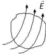
Рис. 27. Поток векторной функции через замкнутую поверхность произвольной формы (случай плоскости)
