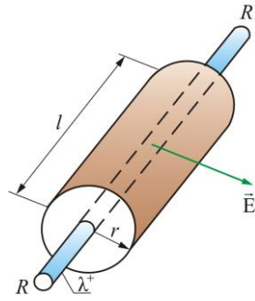
Рис. 29. К вычислению напряженности поля, создаваемого бесконечной равномерно заряженной нитью
