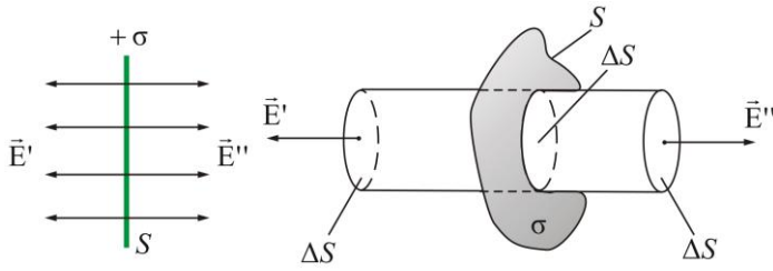
Рис. 28. Иллюстрация к вычислению напряженности поля, создаваемого бесконечной равномерно заряженной плоскостью
