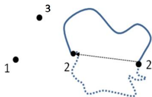
Рис. 11. К нахождению энергии системы зарядов
