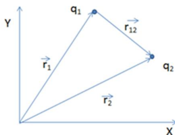
Рис. 4. Напоминание правила вычитания векторов.
