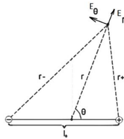
Рис.18. К вычислению потенциала диполя
