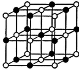
Рис. 12. Гранецентрированная решётка, состоящая из атомов двух сортов.
