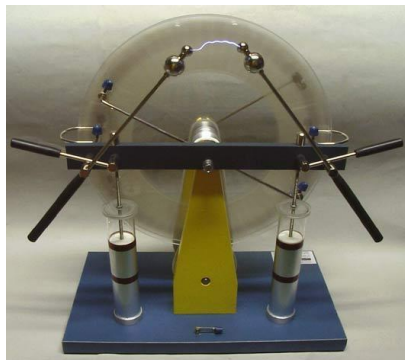
Рис. 1. Электрофорная машина.
