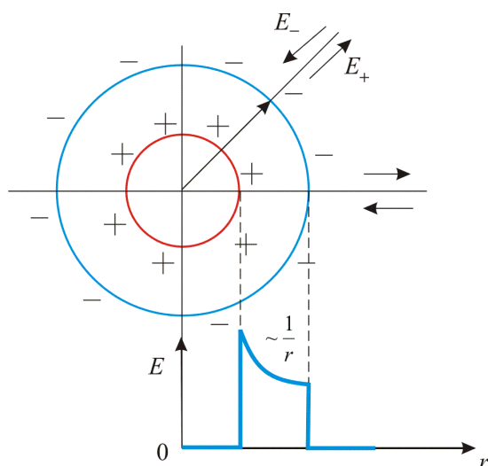
Рис. 30. Зависимость напряженности поля от расстояния для случая равномерно заряженной подповерхности нити конечной толщины.
