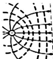
Рис. 15. Пример эквипотенциальной поверхности для случая, показанного рисунком выше. Эквипотенциальные поверхности даны пунктиром
