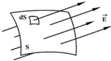
Рис. 23. Пример потока линий ЭП через поверхность произвольной формы
