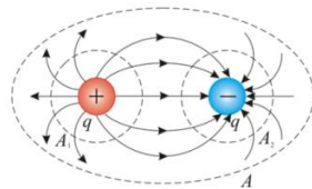
Рис. 24. Поток через различные поверхности, окружающие систему зарядов
