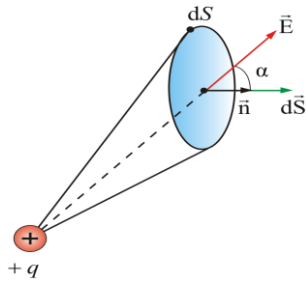
Рис. 25. Расчёт потока через замкнутую поверхность произвольной формы
