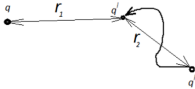
Рис.10. К подсчёту энергии системы зарядов
