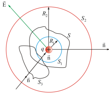
Рис. 26. Вычисление потока через сферическую поверхность
